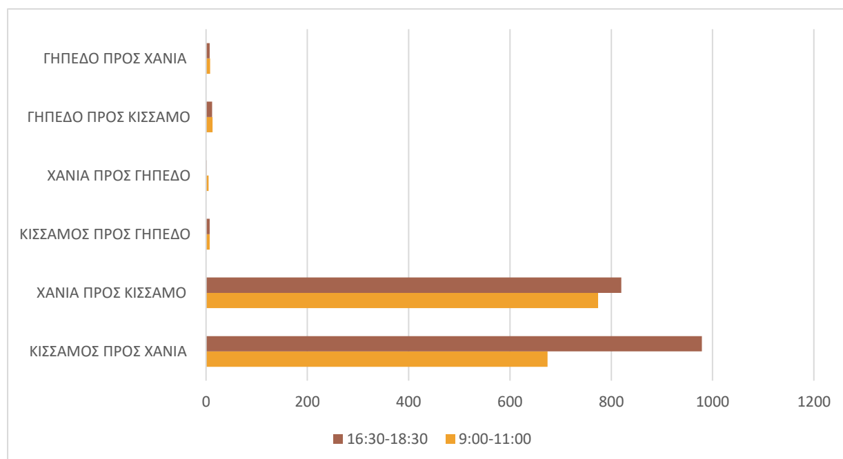
Γράφημα 12: Φόρτοι μετακινήσεων & στρέφουσες μετακινήσεις
